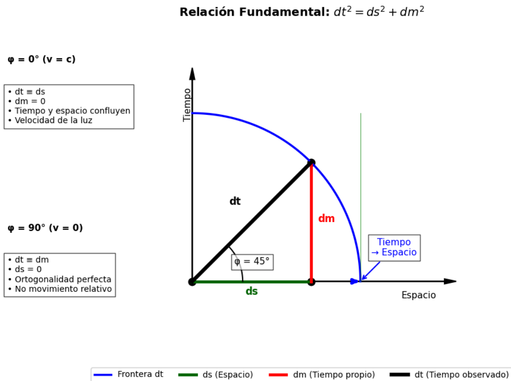
Figure 1: espacio-tiempo
