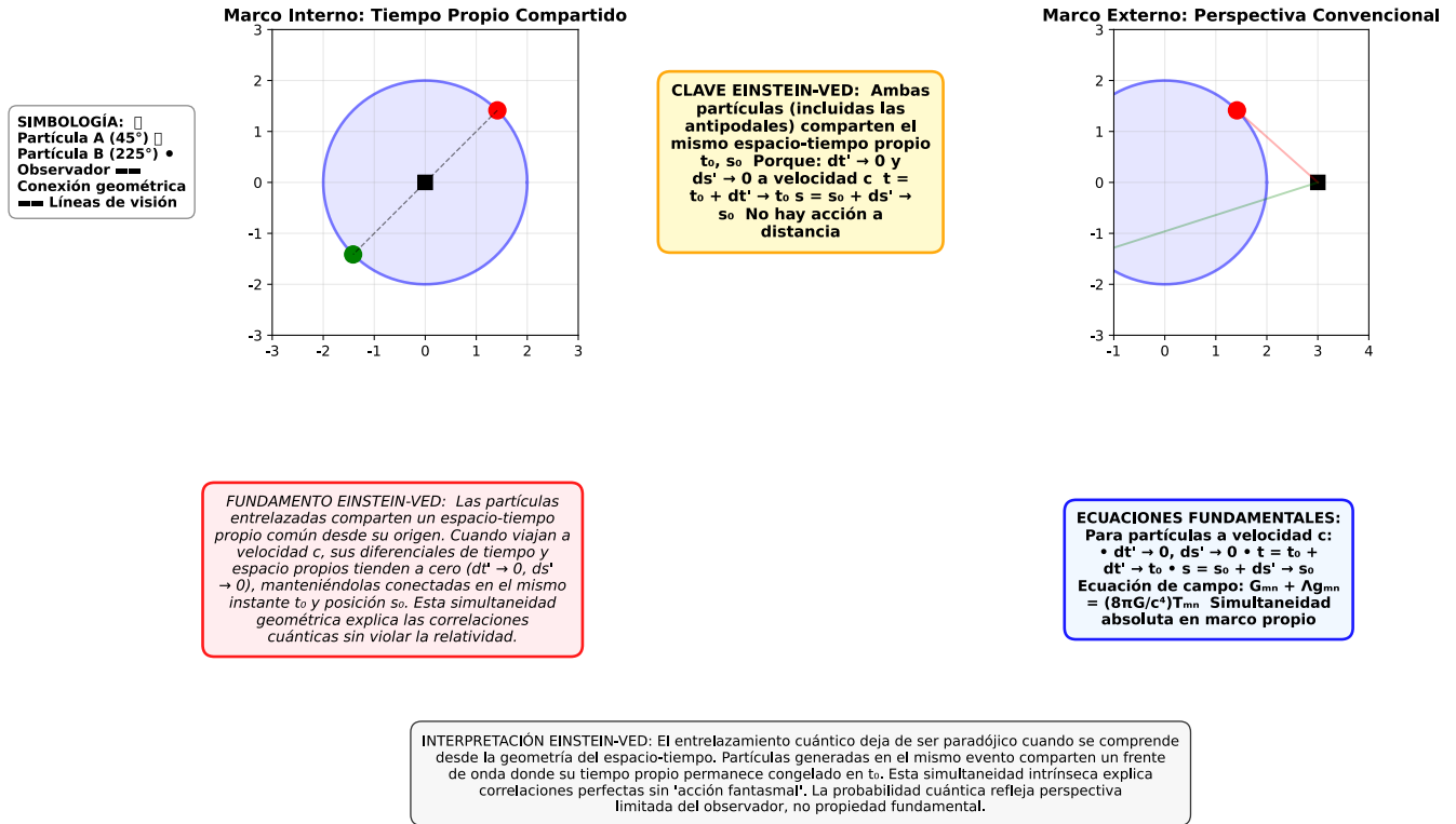
Figura 11: Representación del entrelazamiento cuántico como un modo geométrico compartido entre dos sistemas. En lugar de "acción fantasmal a distancia", los sistemas entrelazados comparten un único número cuántico n global, lo que explica sus correlaciones sin violar localidad.
