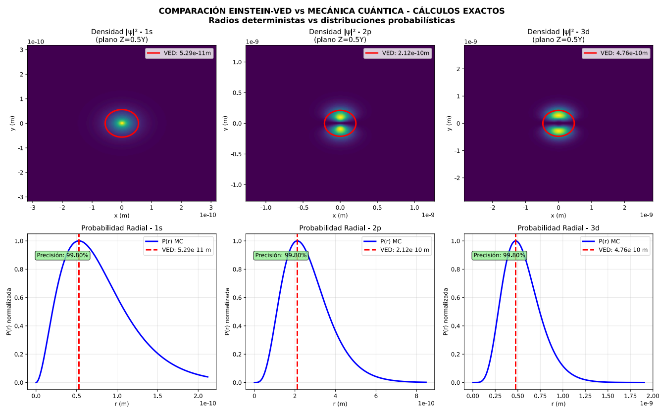
Figura 10: Comparación conceptual - Enfoque geométrico determinista vs probabilístico
