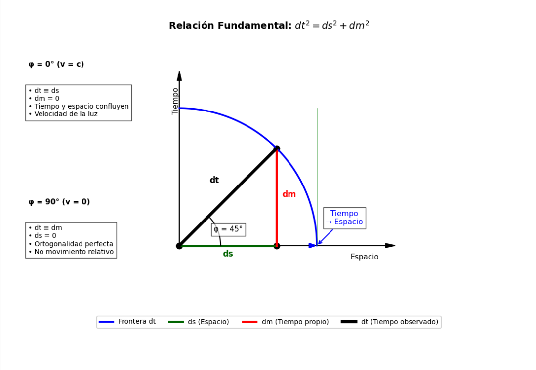
Figure 1: espacio-tiempo
