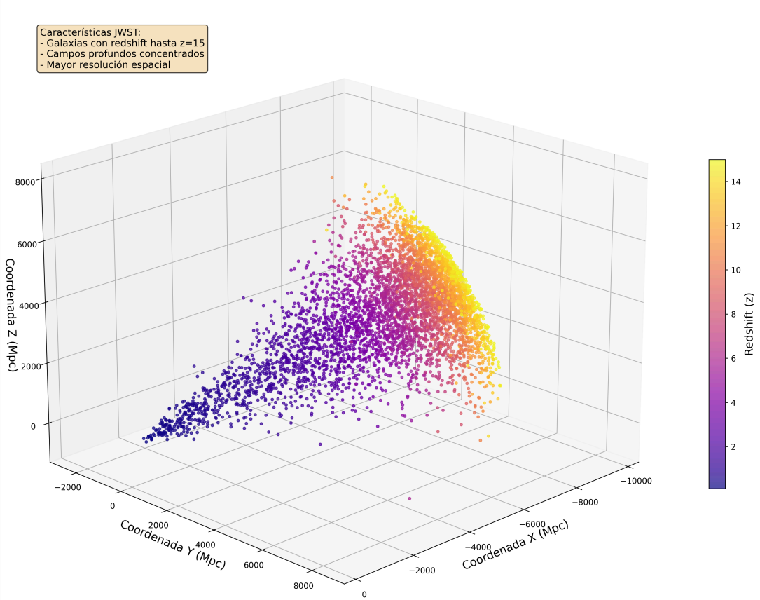
Distribución 3D de 5000 Galaxias - Datos JWST (Simulación)
